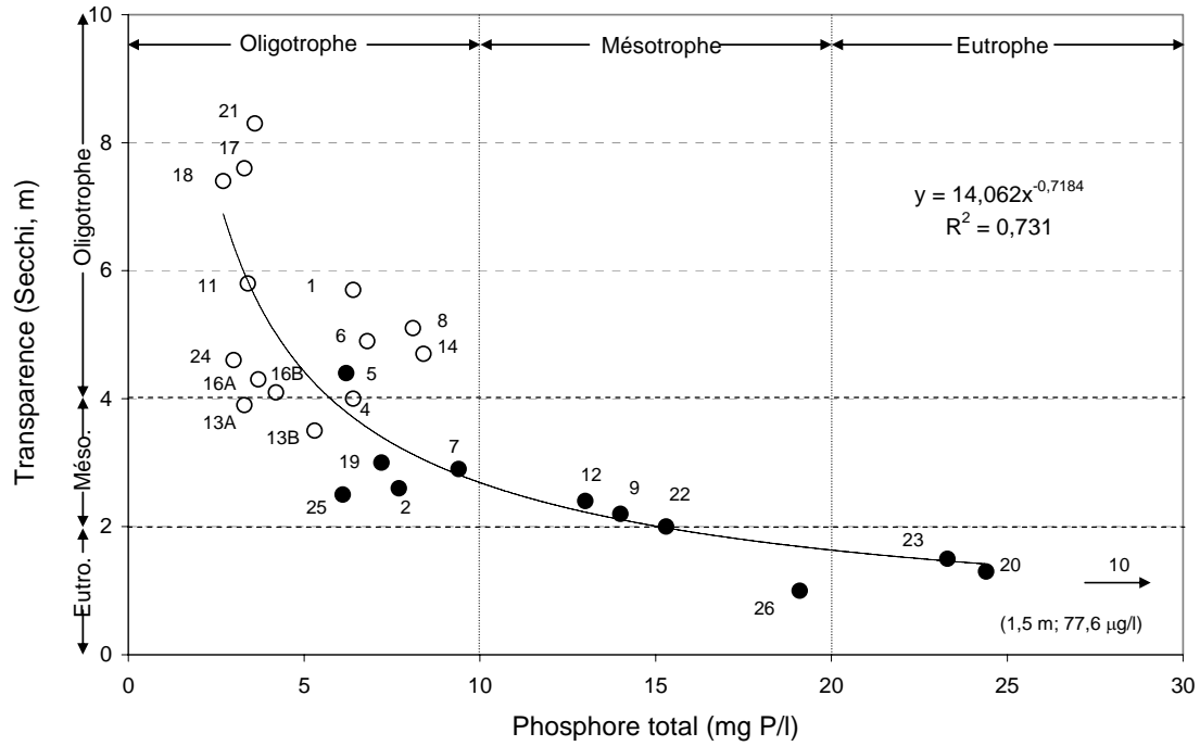
Figure 5 Évaluation du niveau trophique à l'aide de la relation transparence – phosphore total établie à partir des données de la campagne estivale 2003. Les lacs sont identifiés par leur numéro. Cercle noir = COD > 5 mg/l
